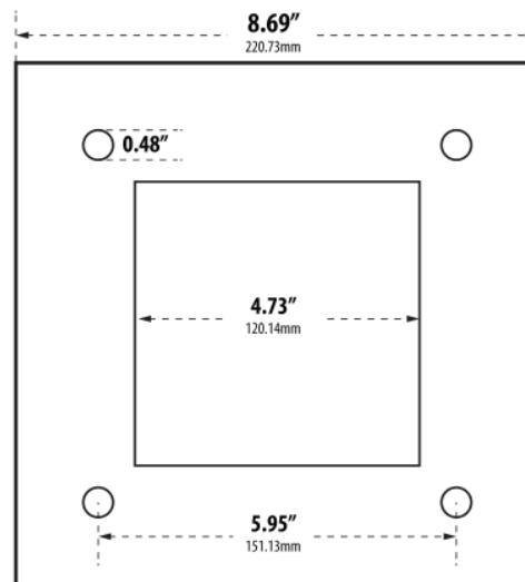
TEMPLATE PATTERN
