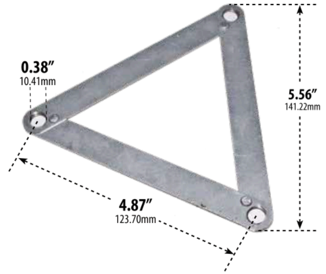
TEMPLATE PATTERN
