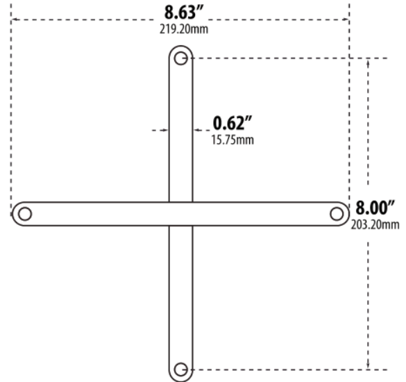
TEMPLATE PATTERN
